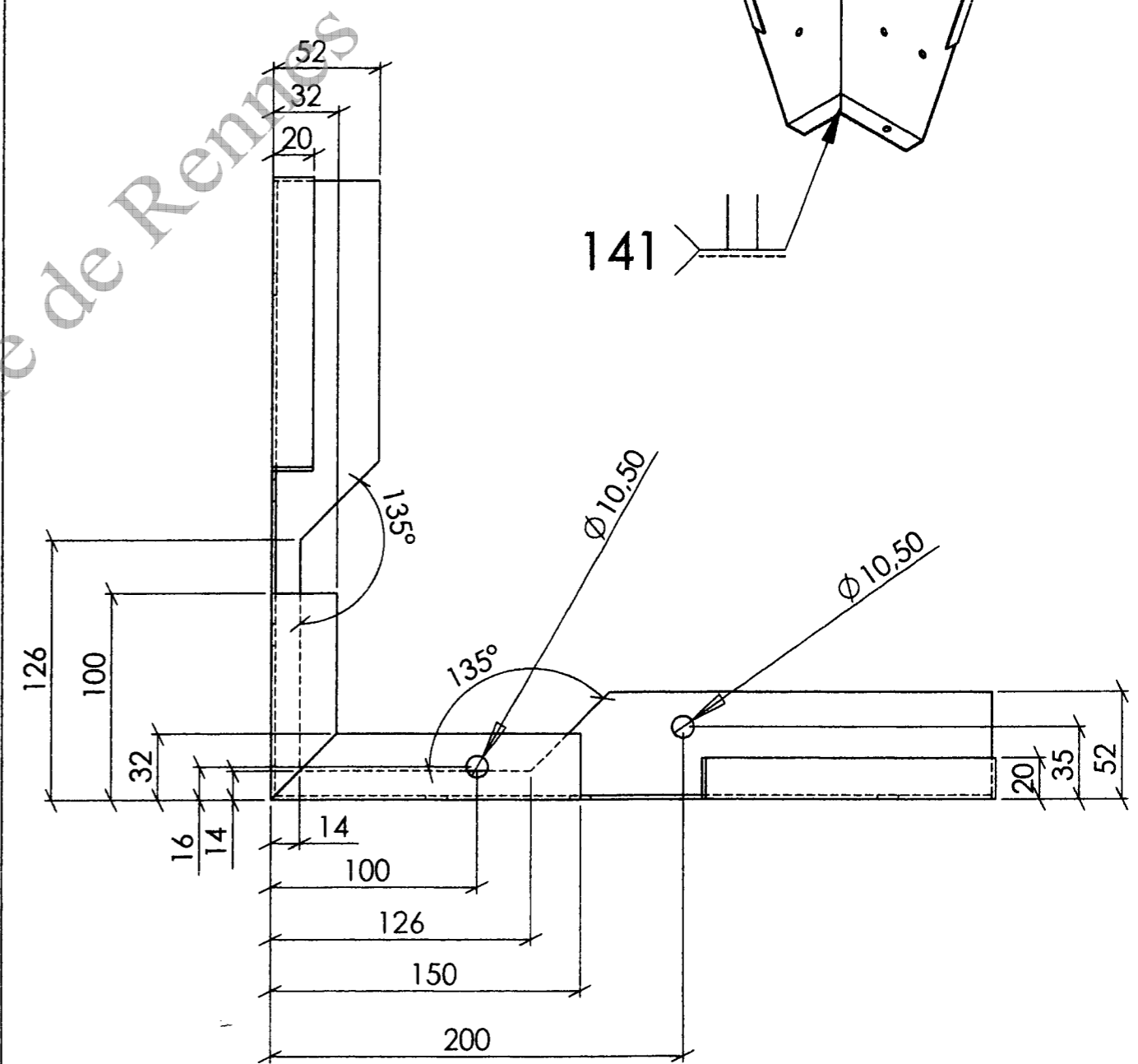
Détail de la vue de dessous à l'échelle 1/3
