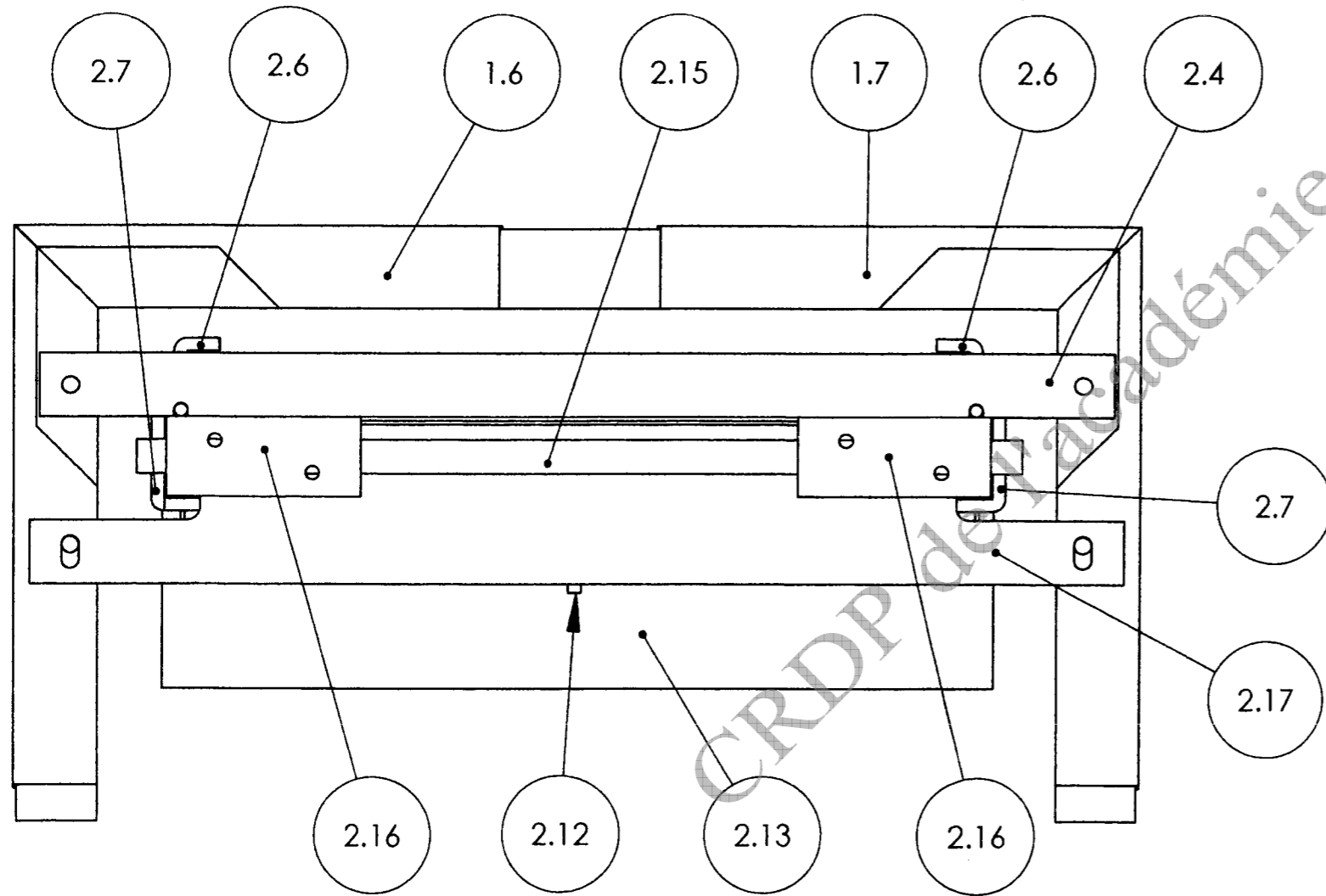
Détail A
