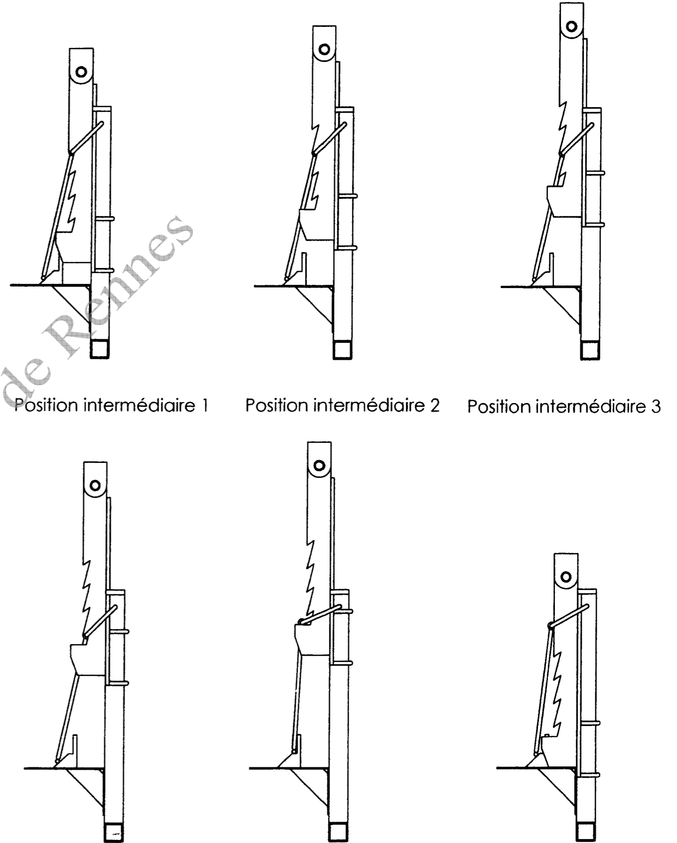
Ensemble 2 principe de fonctionnement
